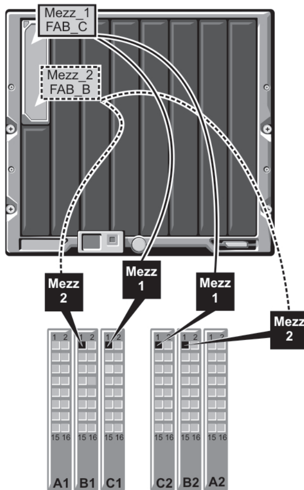
Figure 17. Exemple d'adressage de ports pour un serveur lame mi-hauteur
