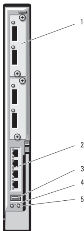
Figure 29. Module commutateur d'E/S Ethernet PowerConnect M6220
