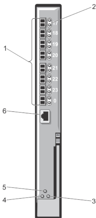
Figure 18. module d'E/S SAN FC 16 Gbps Brocade M6505
