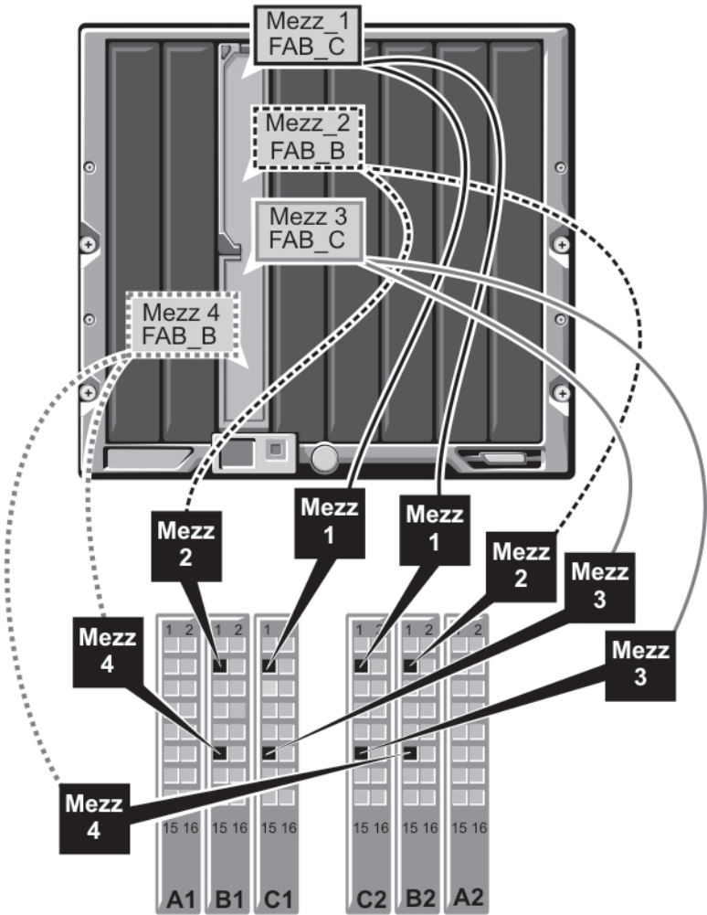
Figure 16. Exemple d'adressage de ports pour serveur lame pleine hauteur – Serveur lame 3 (ne s'applique pas au système PowerEdge M610x)
