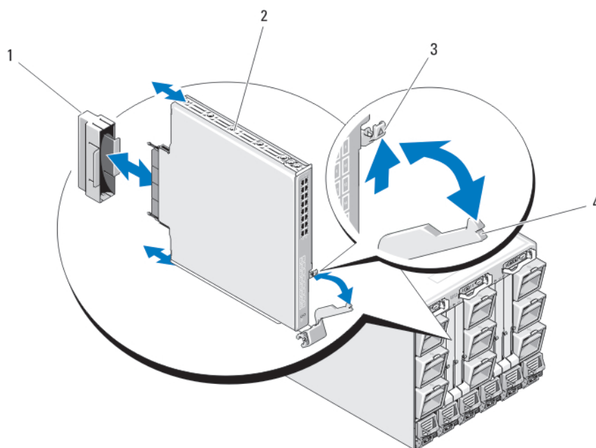
Figure 48. Retrait et installation d'un module d'E/S
