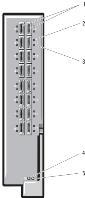
Figure 26. Module commutateur d'E/S Mellanox M3601Q QDR Infiniband
