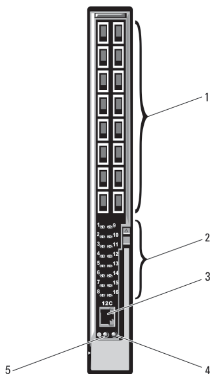
Figure 22. Module du commutateur Mellanox M4001F/M4001Q/M4001T Infiniband
