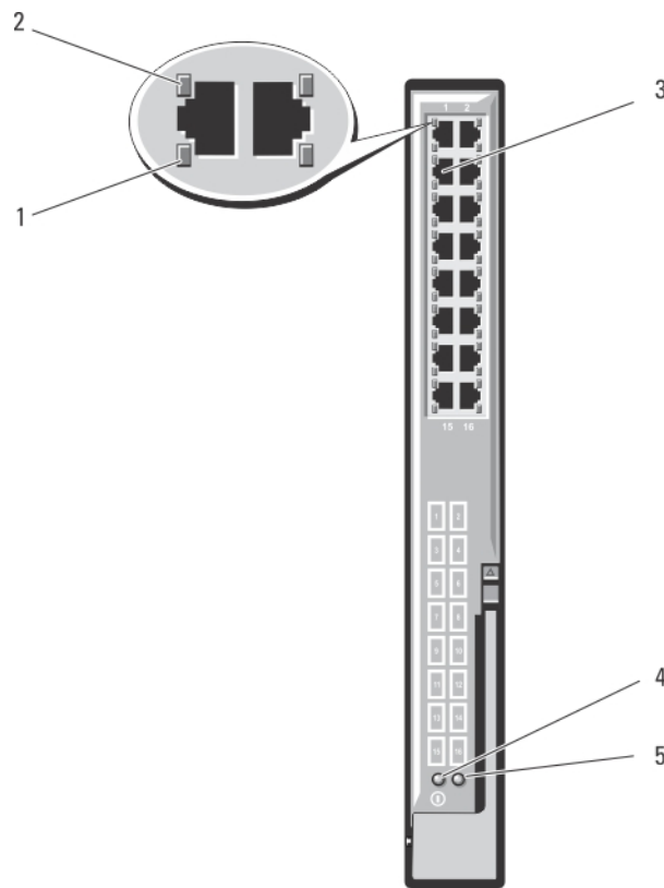
Figure 36. Module d'intercommunication d'E/S Ethernet 10/100/1 000 Mbit
