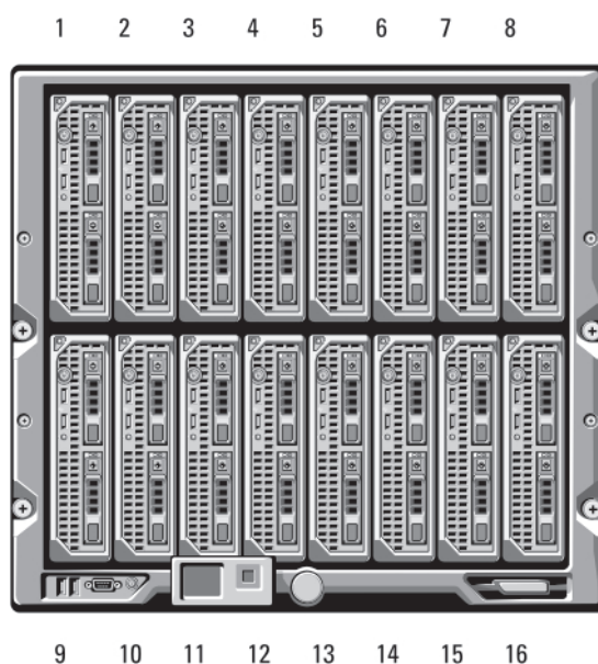
Figure 1. Numérotation des serveurs lames : serveurs lames mi-hauteur
