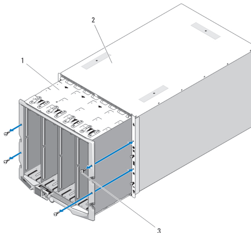
Figure 50. Retrait et installation du bâti des modules avant
