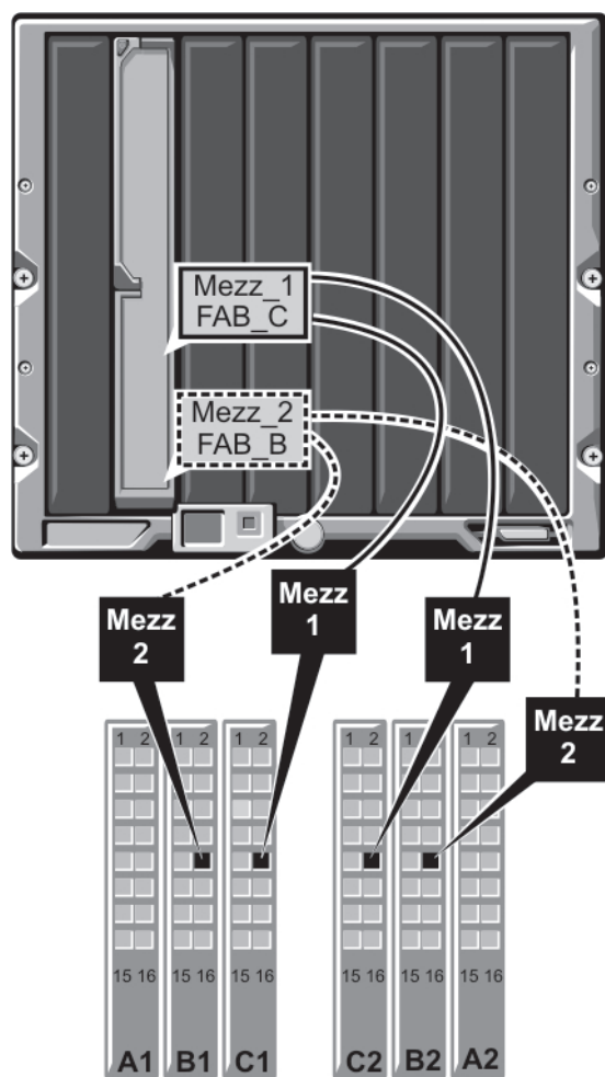
Figure 15. Exemple d'adressage de ports pour un système PowerEdge M610x – Serveur lame 2
