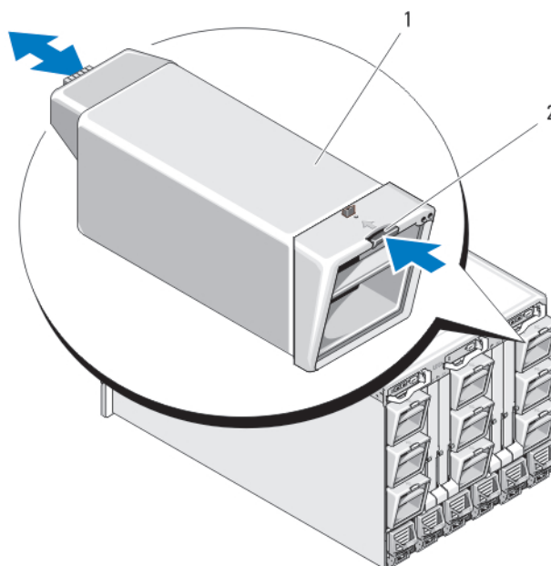
Figure 44. Retrait et installation d'un module de ventilation
