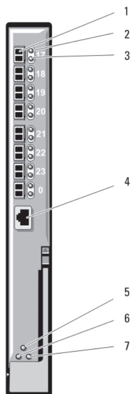
Figure 32. Module d'E/S Brocade M5424 pour réseau FC8
