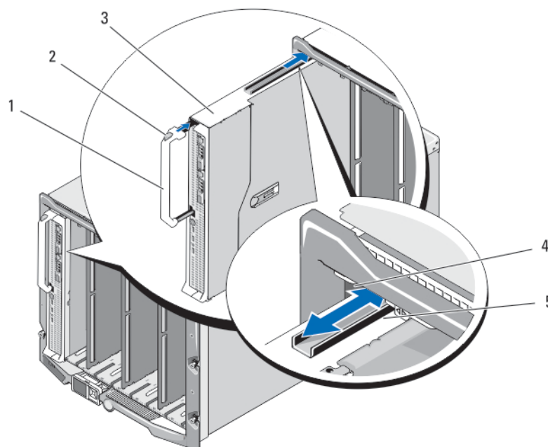
Figure 38. Retrait et installation d'un serveur lame pleine hauteur
