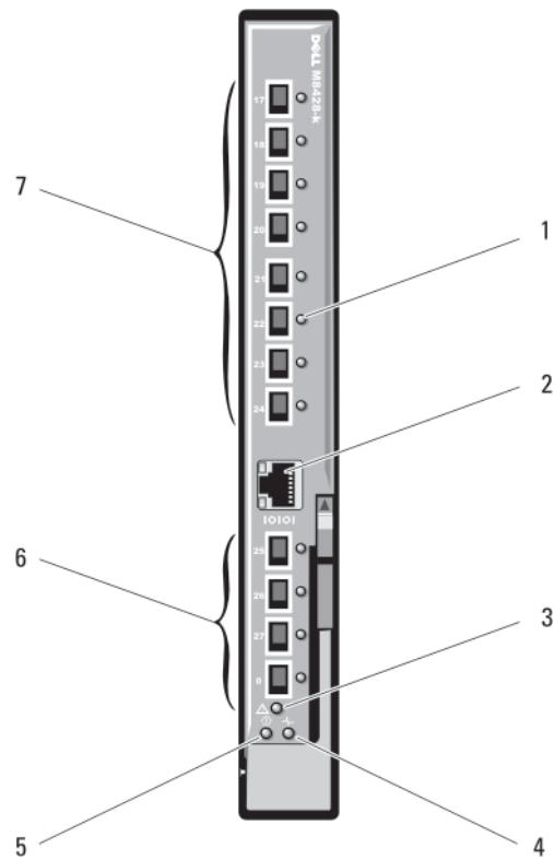
Figure 24. Commutateur réseau convergé 10 Gbit Dell PowerConnect M8428-k
