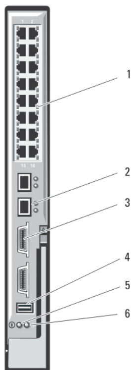
Figure 28. Fonctionnalités du module commutateur d'E/S Ethernet 1 Gbit PowerConnect M6348
