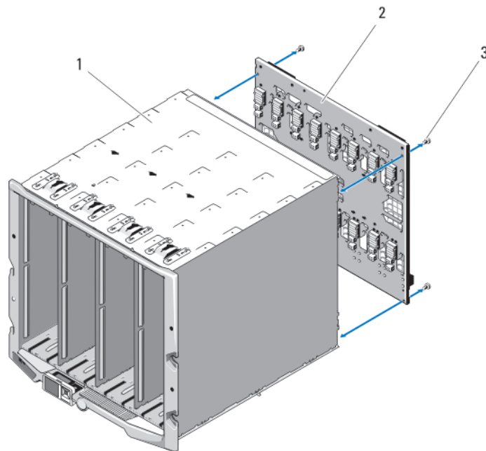
Figure 51. Retrait et installation du fond de panier central
