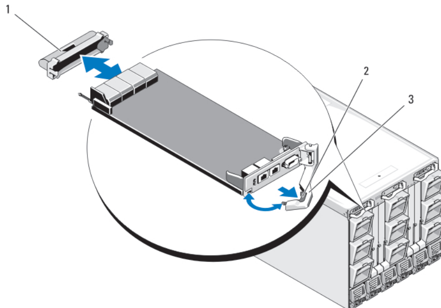
Figure 47. Retrait et installation d'un module CMC ou d'un module iKVM (module CMC représenté)
