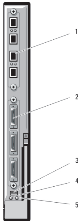
Figure 30. Module commutateur d'E/S Ethernet PowerConnect M8024 10 Gbit
