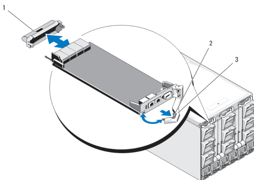
Figure 45. Retrait et installation d'un module CMC ou d'un module iKVM (module CMC représenté)
