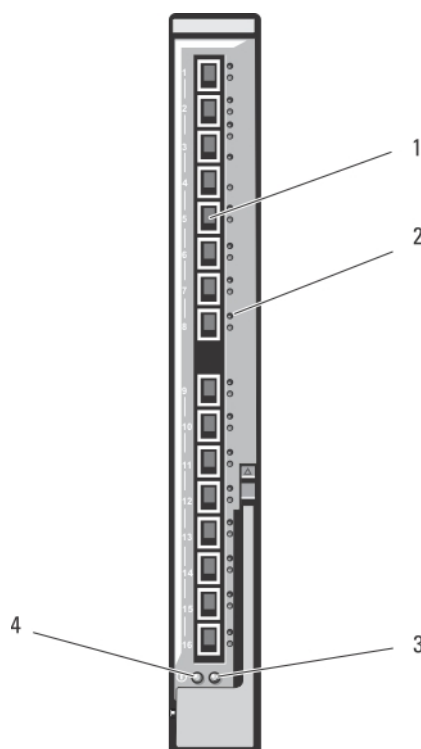
Figure 34. Module d'intercommunication 10 GbE KR Dell
