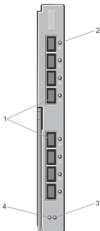
Figure 19. Module d'extenseur de matrice B22 Cisco Nexus
