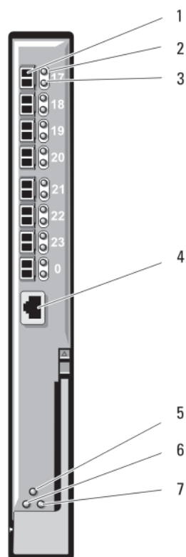
Figure 31. Module Fibre Channel 8/4 Gbit/s Dell pour réseau SAN
