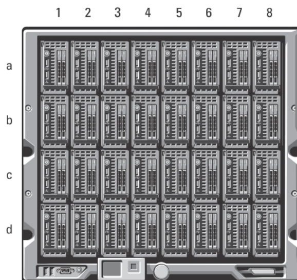
Figure 3. Numérotation des serveurs lames : serveurs lames quarter-height
